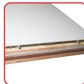
Zavírání - dvoubodové zasouvací čepy
